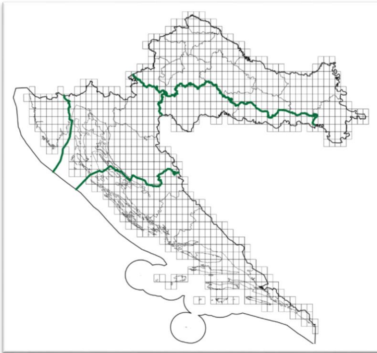
Slika 2. Mreža EMEP modela na skali 0.1° x 0.1° (8 km x 11 km) raspoređena po teritoriju RH
