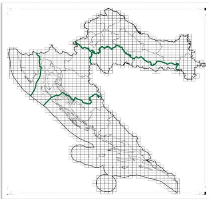
Slika 3. Mreža LOTOS-EUROS modela na skali 0.125° x 0.0625° (10 km x 7 km) raspoređena po teritoriju RH
