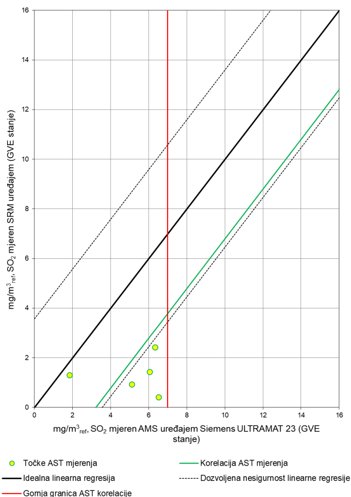
Sl. 12: Odnos utvrđene AST korelacije i idealnog regresijskog pravca AMS uređaja Siemens ULTRAMAT 23 za mjerenje SO 2 u suhim dimnim plinovima
