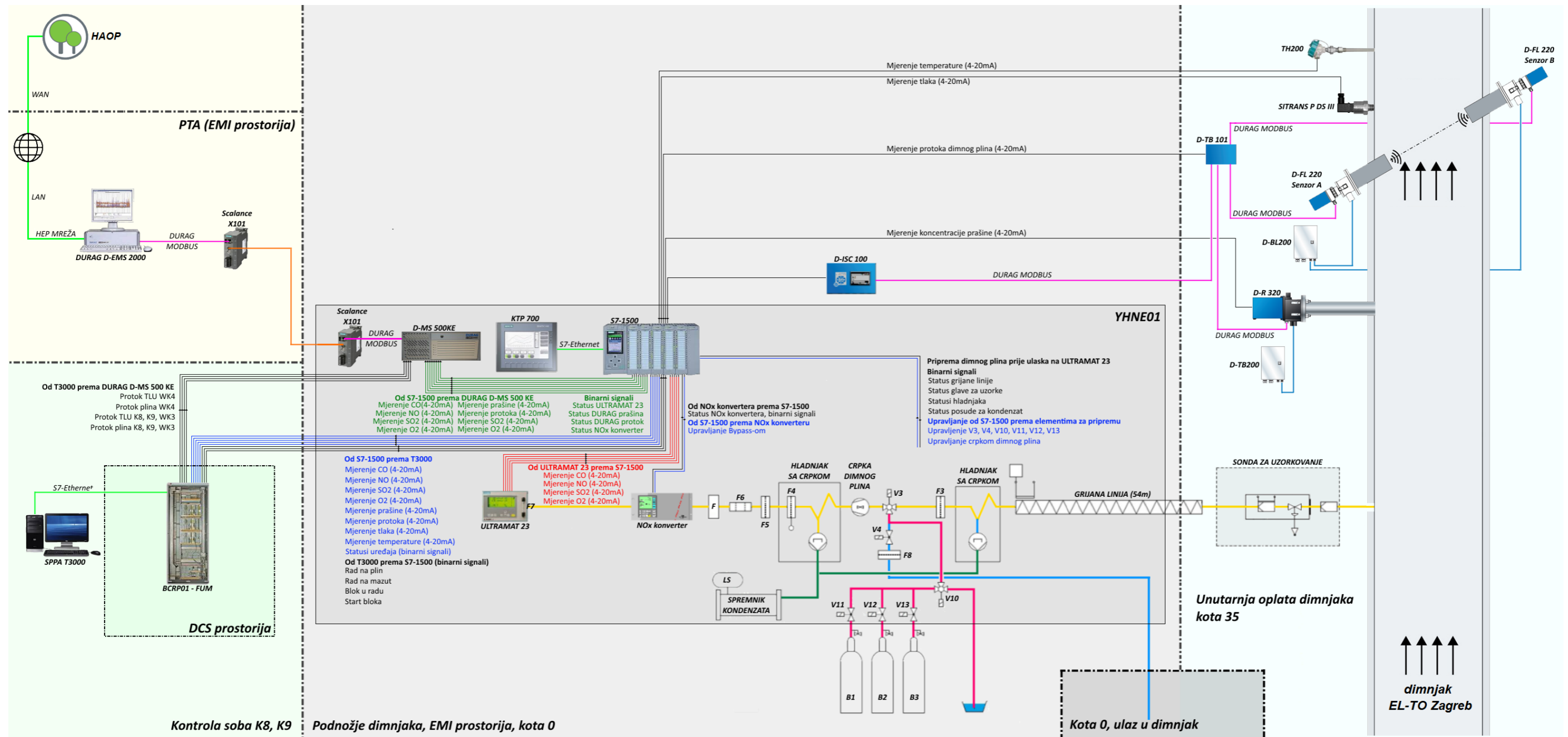
Sl. 2: Shematski prikaz automatskog mjernog sustava glavnog dimnjaka EL-TO Zagreb
