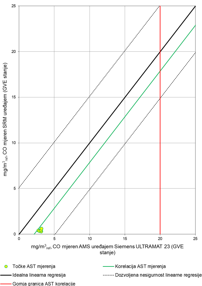
Sl. 13: Odnos utvrđene AST korelacije i idealnog regresijskog pravca AMS uređaja Siemens ULTRAMAT 23 za mjerenje CO u suhim dimnim plinovima
