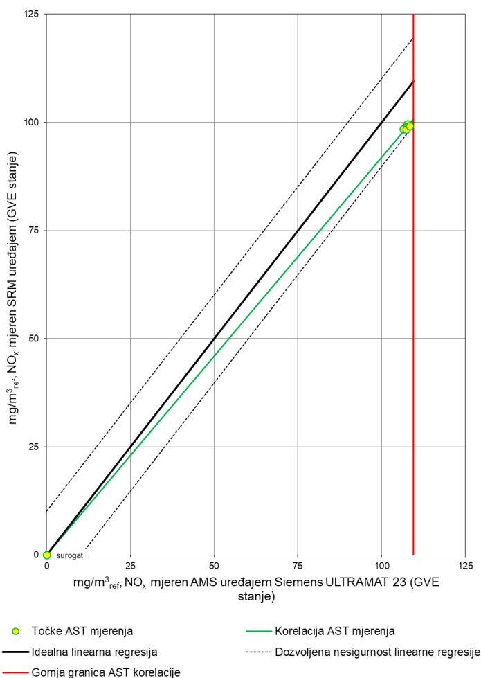
Sl. 11: Odnos utvrđene AST korelacije i idealnog regresijskog pravca AMS uređaja Siemens ULTRAMAT 23 za mjerenje NO x u suhim dimnim plinovima
