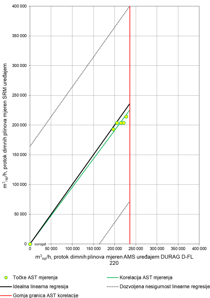
Sl. 15: Odnos utvrđene AST korelacije i idealnog regresijskog pravca AMS uređaja DURAG D-FL 220 za mjerenje brzine i protoka dimnih plinova
