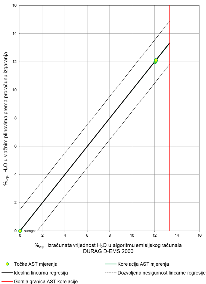
Sl. 9: Odnos utvrđene AST korelacije i idealnog regresijskog pravca za izračunatu vlažnost dimnih plinova
