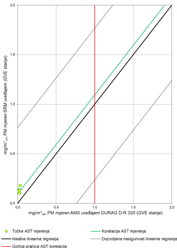
Sl. 14: Odnos utvrđene AST korelacije i idealnog regresijskog pravca AMS uređaja DURAG D-R 320 za mjerenje PM
