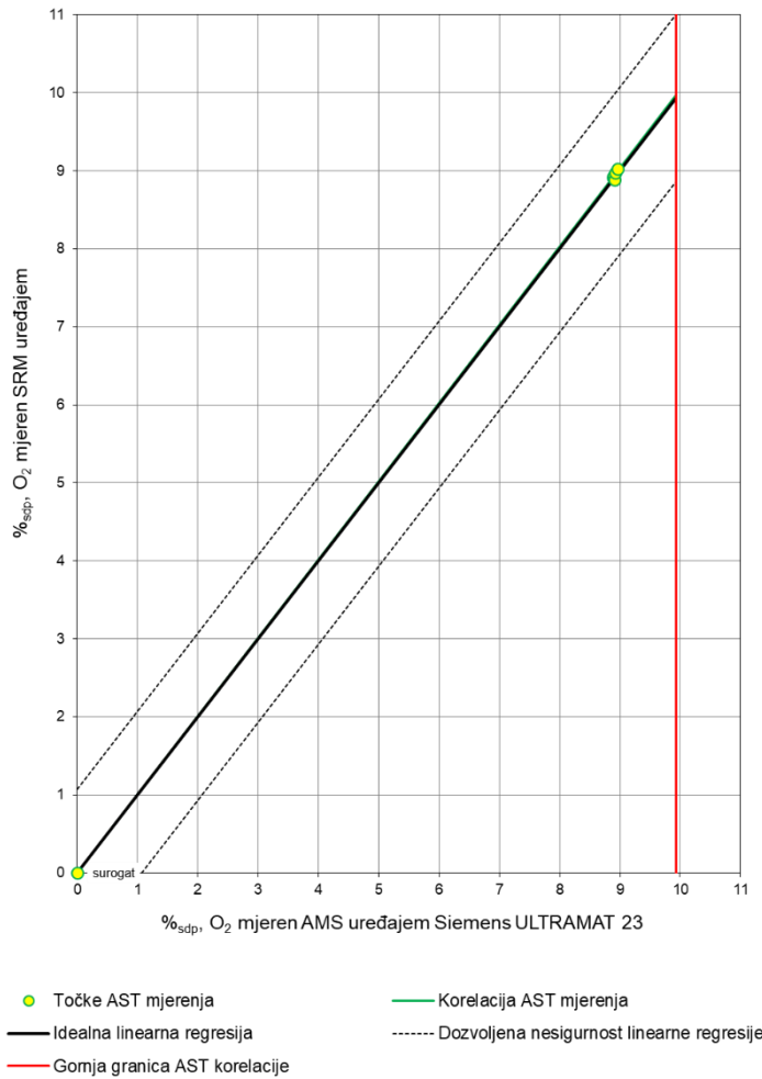
Sl. 10: Odnos utvrđene AST korelacije i idealnog regresijskog pravca AMS uređaja Siemens ULTRAMAT 23 za mjerenje O 2 u suhim dimnim plinovima
