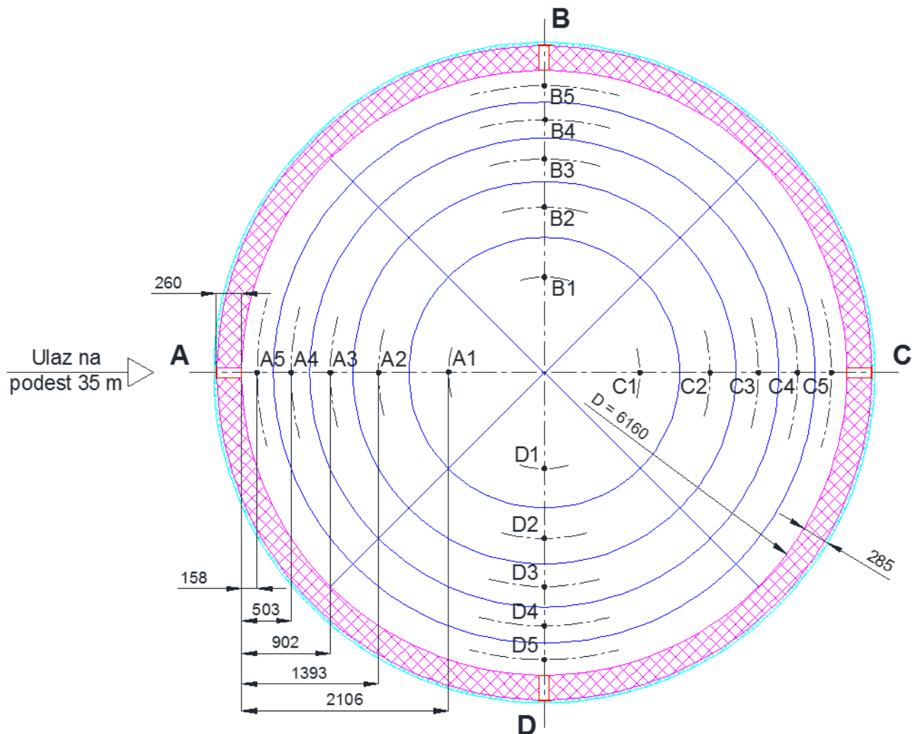
Sl. P 3: Dimenzije i predloženi raspored mjernih točki po mjernom presjeku glavnog betonskog dimnjaka na koti 35 m
