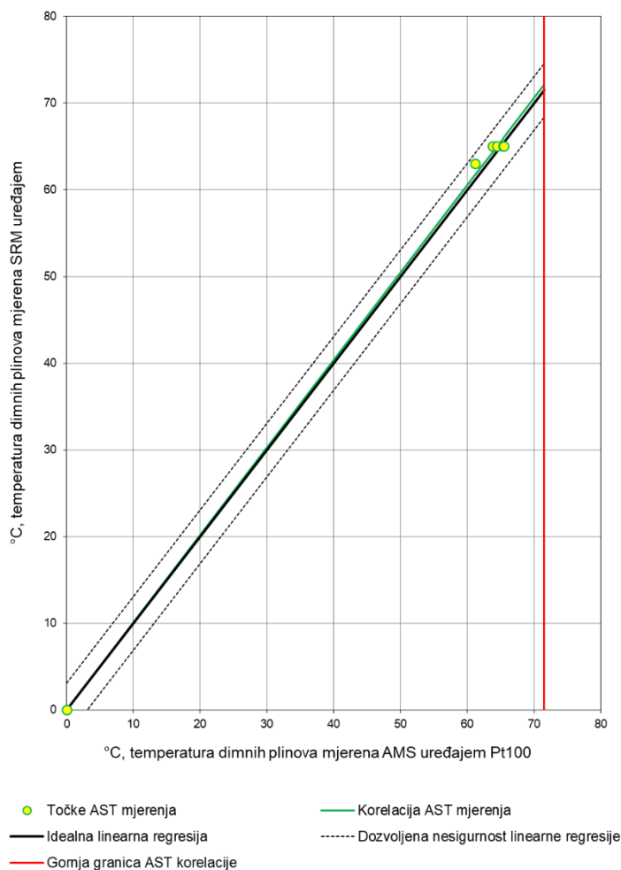
Sl. 7: Odnos utvrđene AST korelacije i idealnog regresijskog pravca AMS uređaja Pt100 za mjerenje temperature
