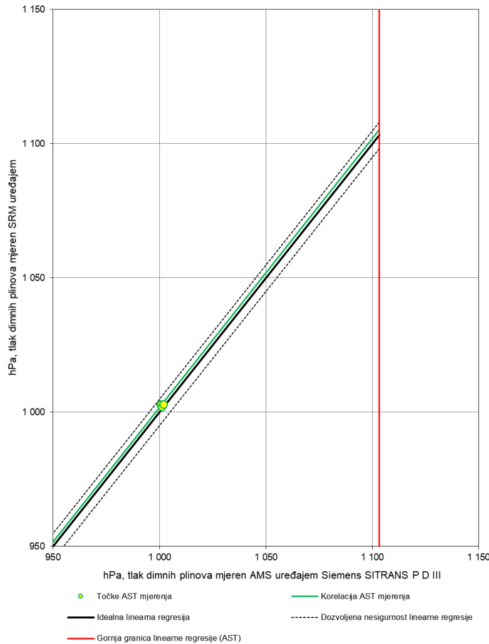
Sl. 8: Odnos utvrđene AST korelacije i idealnog regresijskog pravca AMS uređaja Siemens SITRANS P DS III za mjerenje tlaka
